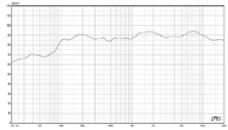
Diagram frequentiereactie:
