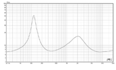
Impedantiediagram:
